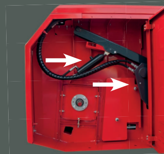
Мотовило настраивается гидравлически по высоте и имеет гидропривод.
