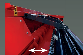
Пропускная способность жатки настраивается гидравлически во время движения.
